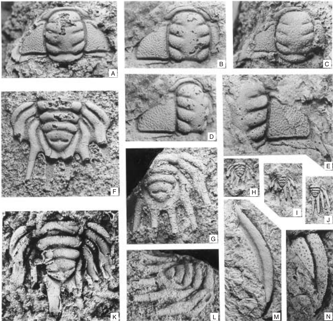
Text-fig. 17. Anacheirurus nanus (MERGL, 1994).
