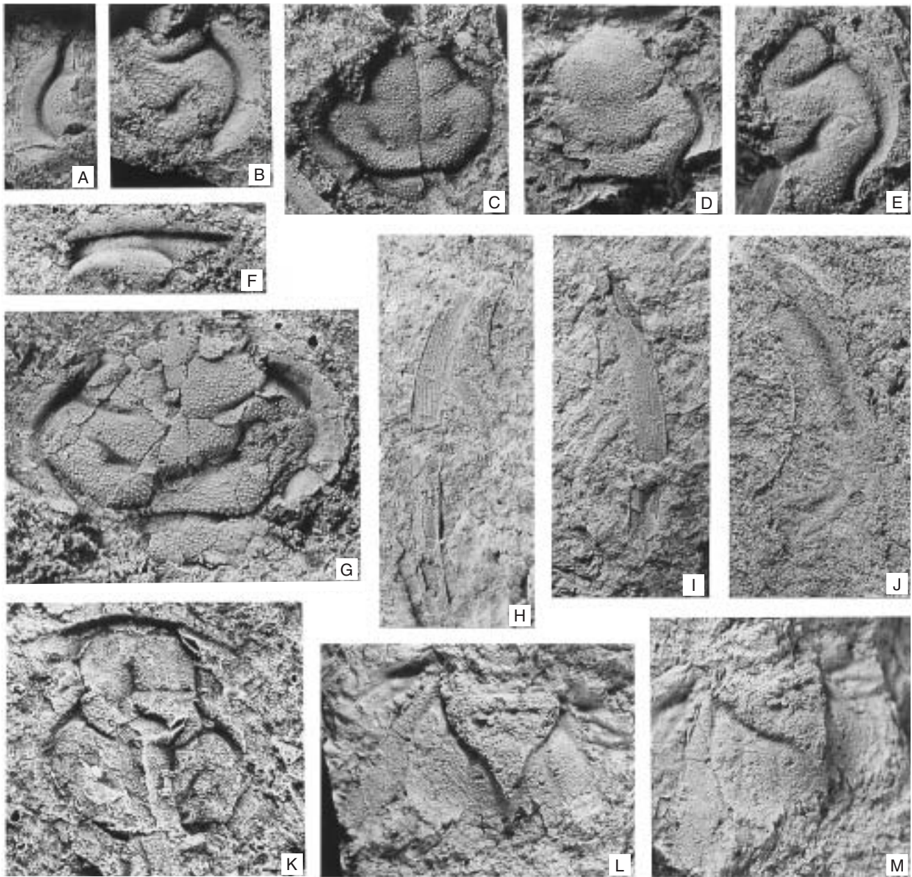
Text-fig. 33. Apatokephalus aff. dagmarae MERGL, 1984.
