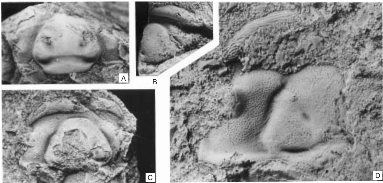
Text-fig. 41. Eulomina mitratum (RŮŽIČKA, 1926).
