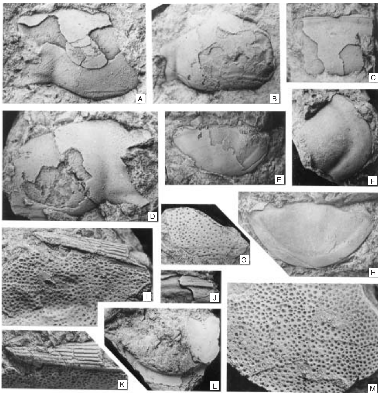
Text-fig. 11. Hemibarrandia holoubkovensis (RŮŽIČKA, 1926).
