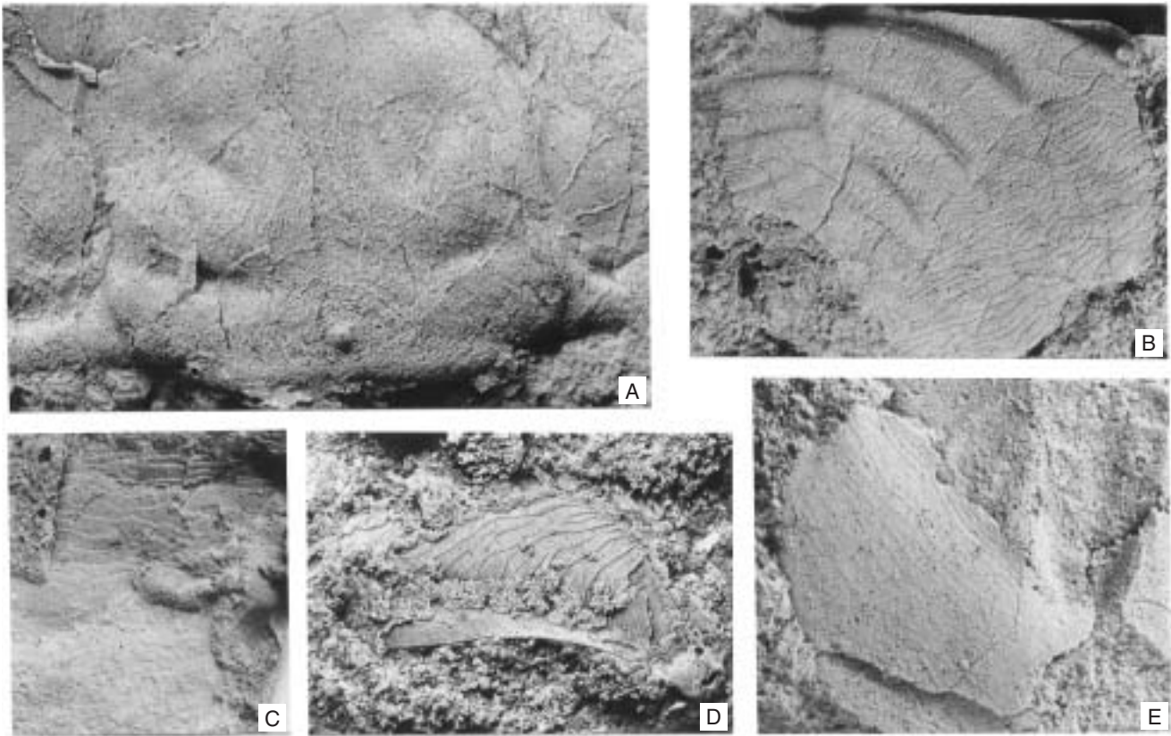
Text-fig. 29. Dikelocephalina ulrichi RŮŽIČKA, 1935.
