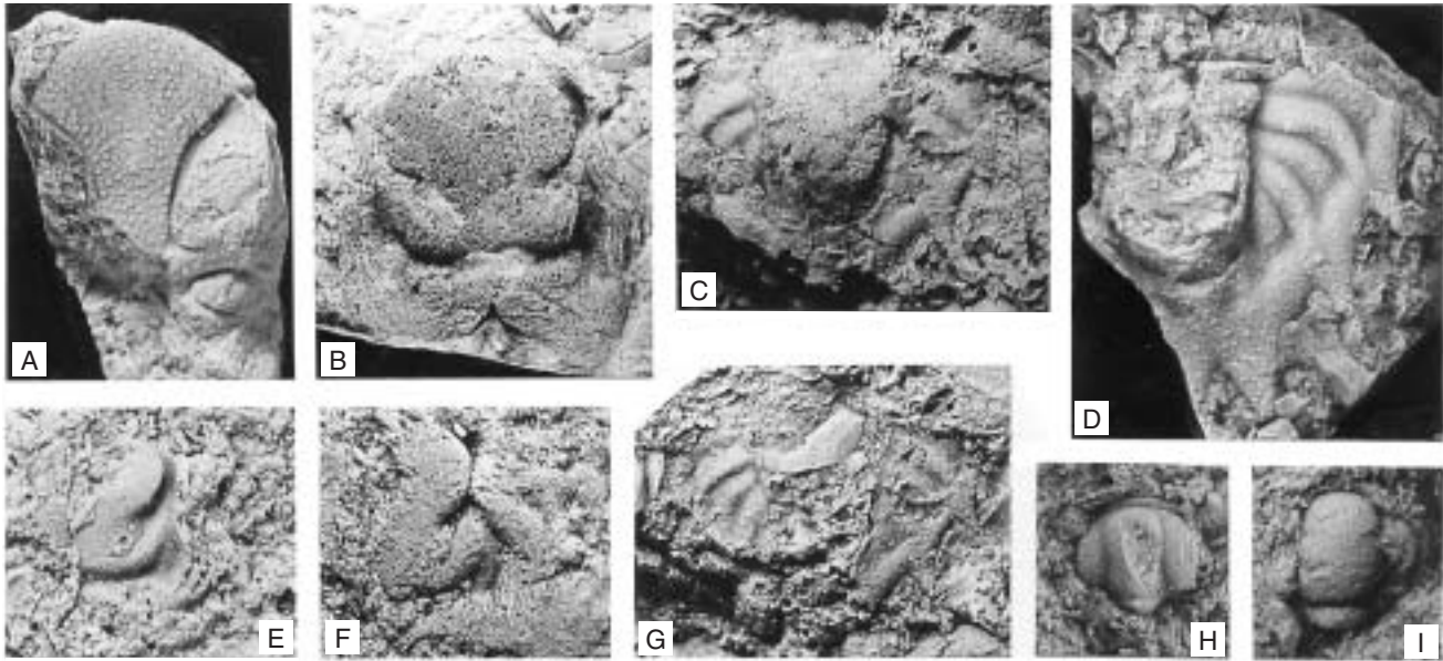
Text-fig. 16. Holoubkovia klouceki (RŮŽIČKA, 1926).
