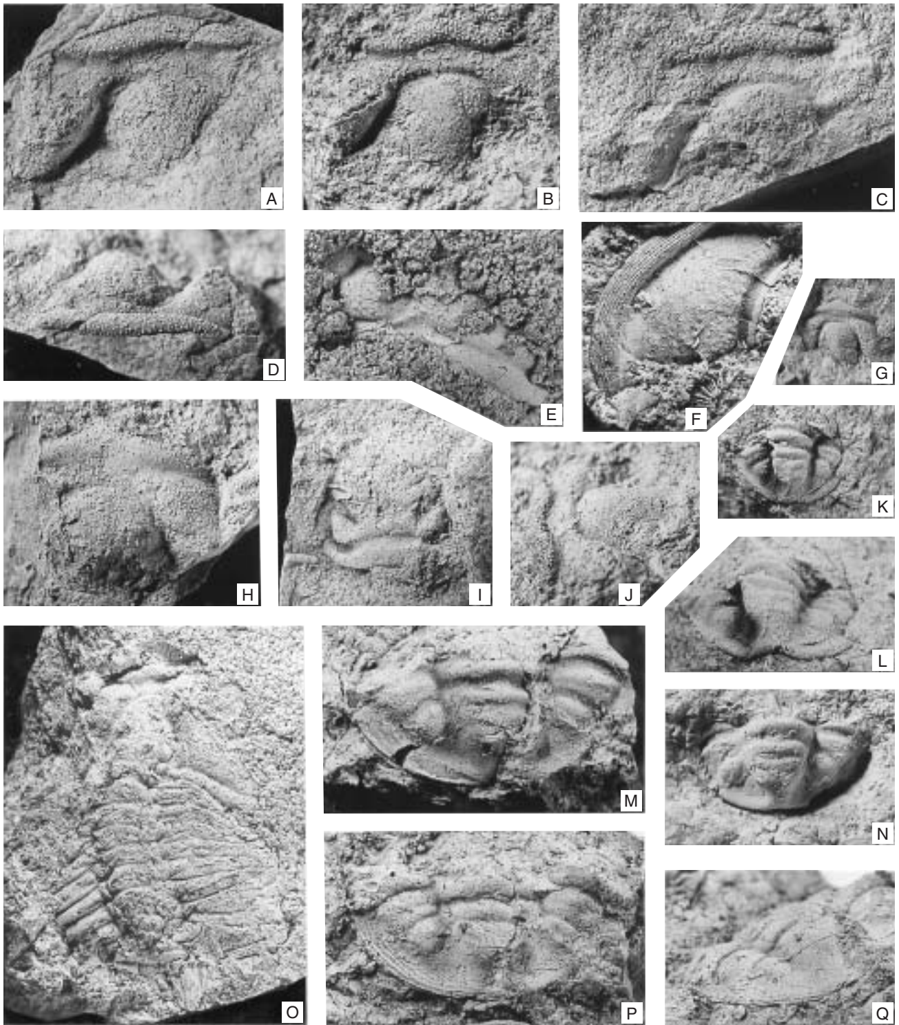
Text-fig. 23. Holoubkocheilus asopus sp. n.
