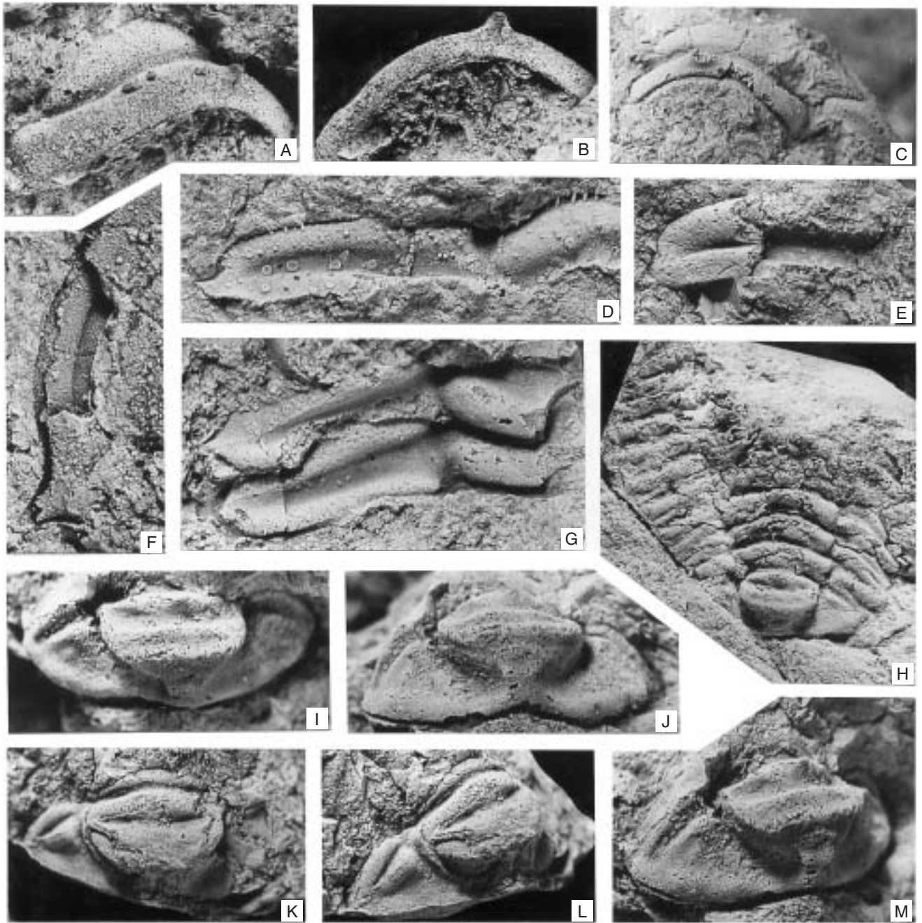
Text-fig. 31. Holubaspis perneri (RŮŽIČKA, 1926).
