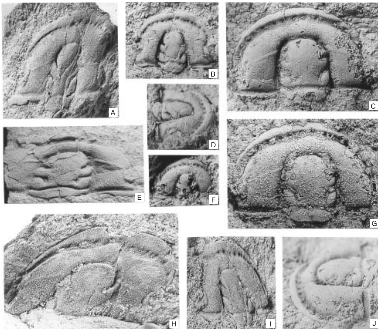
Text-fig. 24. Proteuloma kettneri (RŮŽIČKA, 1941).
