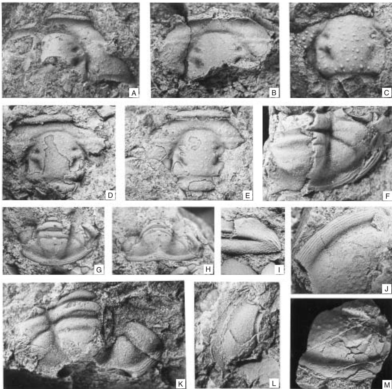
Text-fig. 22. Holoubkocheilus granulatus (RŮŽIČKA, 1926).
