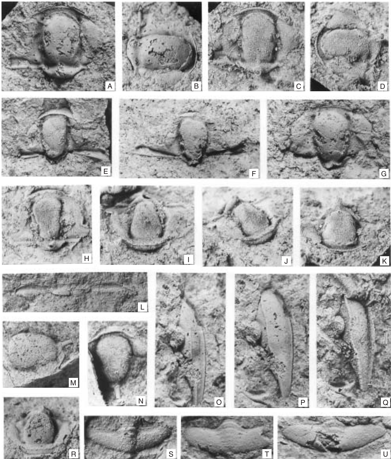
Text-fig. 38. Celdometopus klouceki (VANĚK, 1965).
