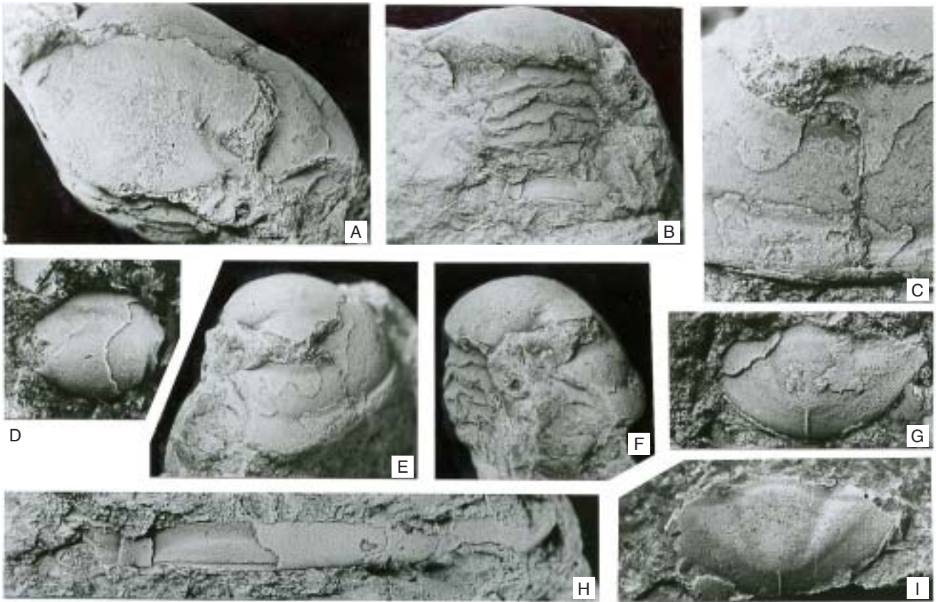
Text-fig. 9. Ottenbyaspis broeggeri (RŮŽIČKA, 1926).
