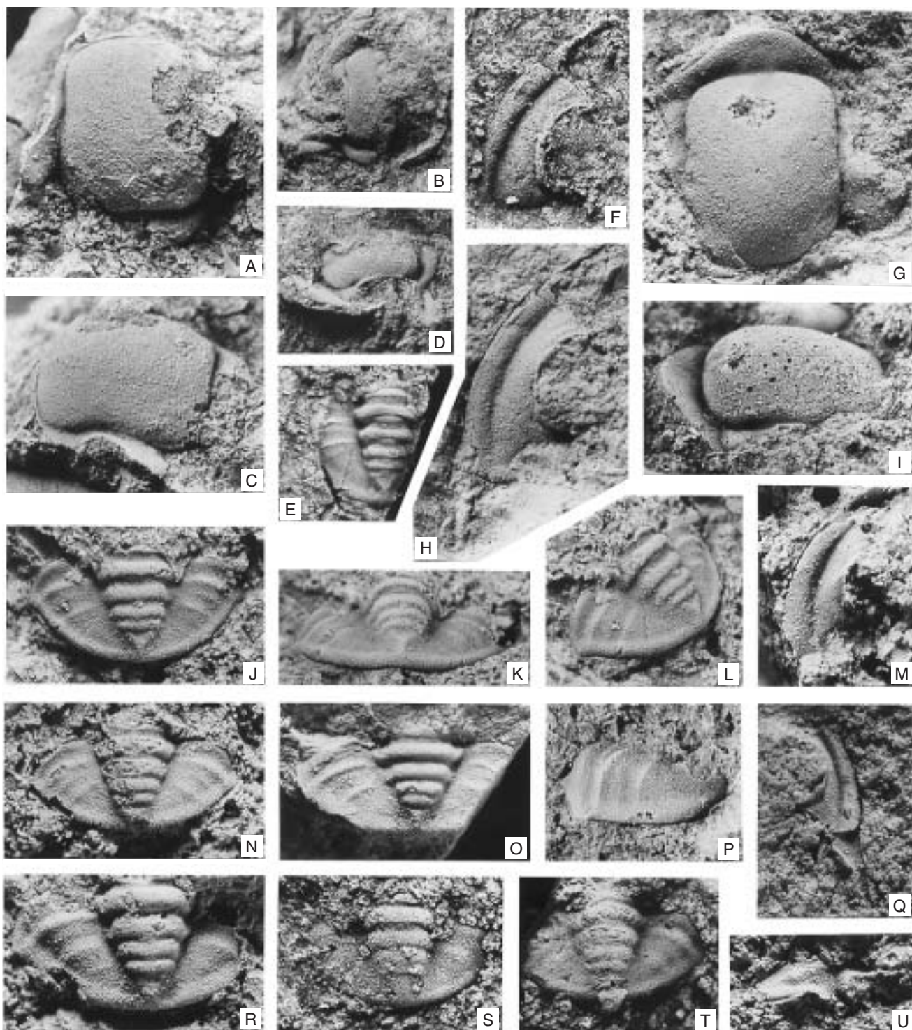
Text-fig. 14. Agerina ferrigena (RŮŽIČKA, 1926).
